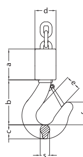
CLW Hook Block 1/1 DIN 15401
