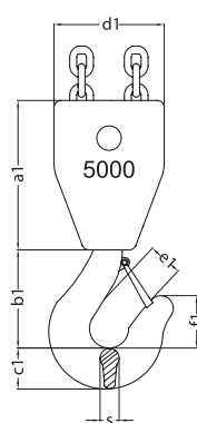
CLW Hook Block 2/1 DIN 15401
